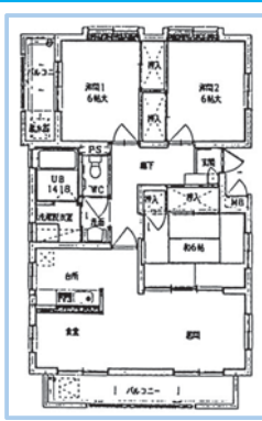
間取り図
