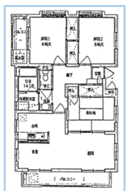
間取り図
